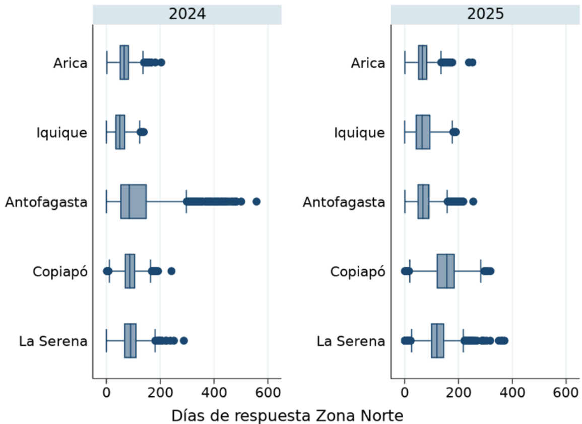
Gráfico N° 1.a Tiempos de respuesta* de solicitudes presentadas por Afiliados a AFP CMR zona norte 2do semestre 2024 y 2do semestre 2025
