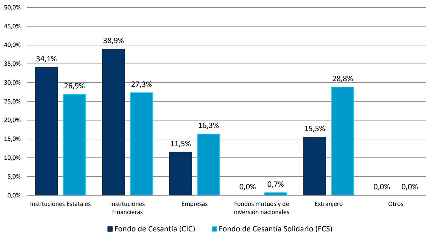
Gráfico N° 3 Diversificación por sector institucional Porcentaje del total de activos al 31 de marzo de 2024
